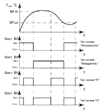
Рисунок 7.1 – Типы логики работы прибора
